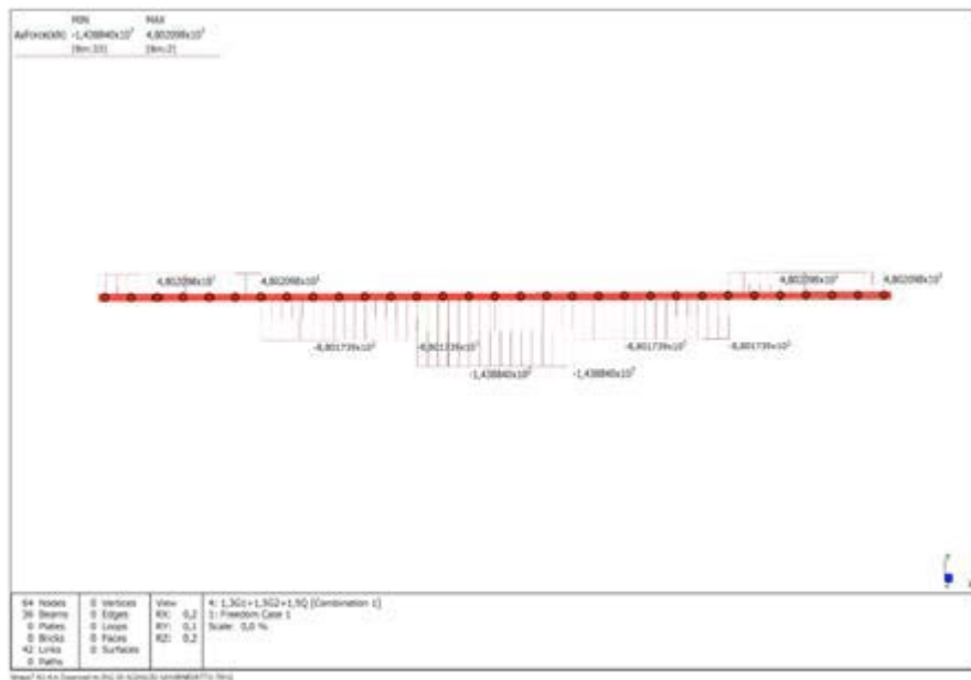
Figura 7. Diagramma dello sforzo normale sulla soletta superiore prodotto dalla combinazione di carico allo SLU 1,3 \cdot G1 + 1,5 \cdot G2 + 1,5 \cdot Q
